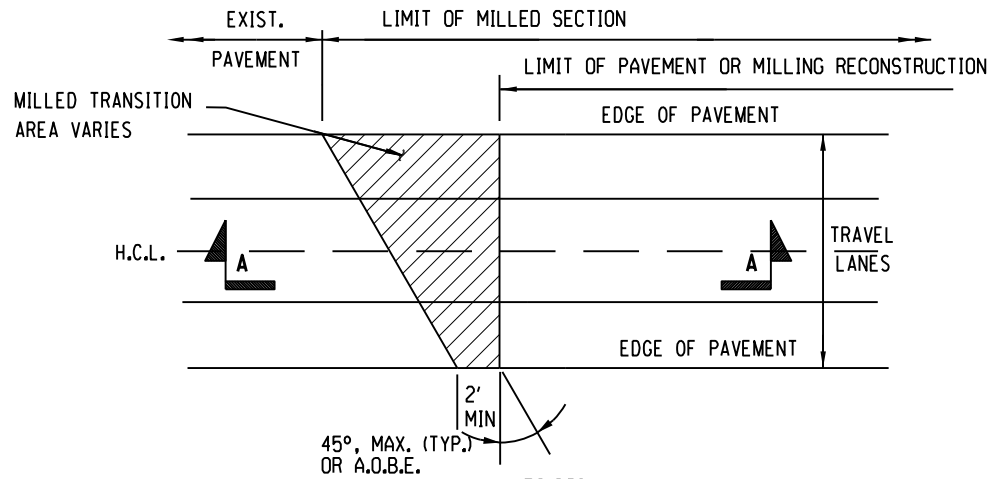
PLAN N.T.S.
