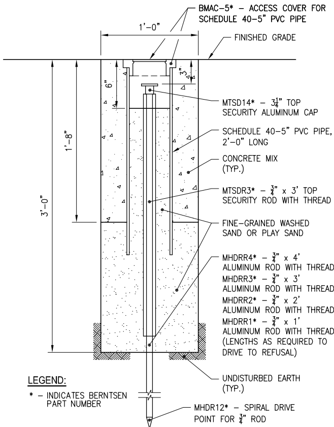
GEODETIC SURVEY MONUMENT N.T.S.
